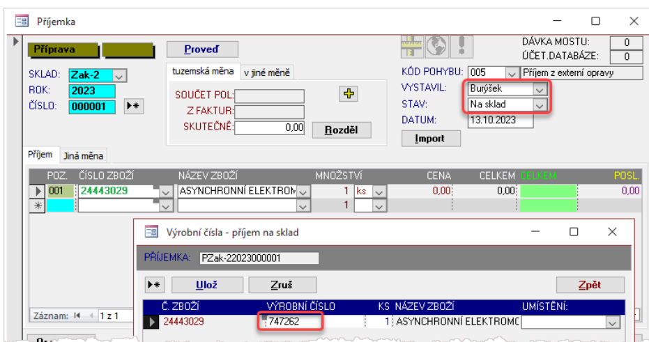
Kompletní Příjemka v systému Soft-4-Sale, připravená k zaskladnění.
